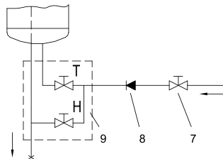
Sl. 4: Otvoreni (protočni) sustav
