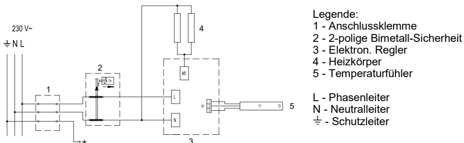
Abb. 6: Elektroschaltbild
